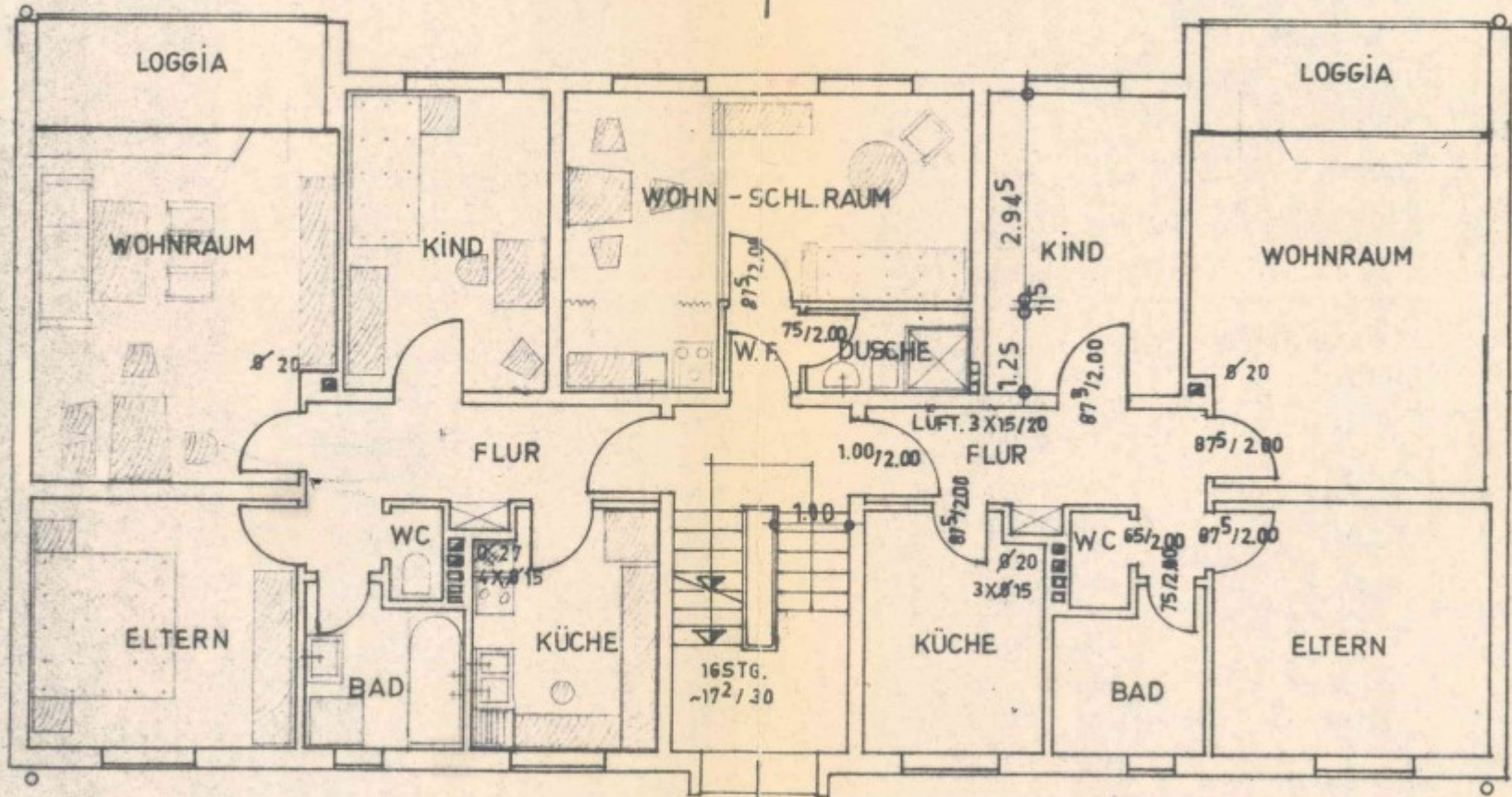
ERD- U. 1. OBERGESCHOSS :
